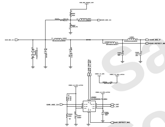
E/J DET IC
