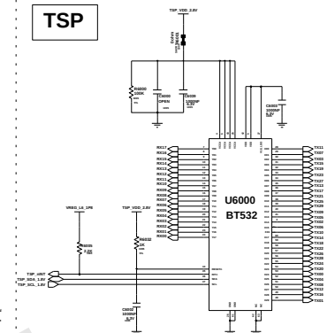
TSP IC (BT532)
