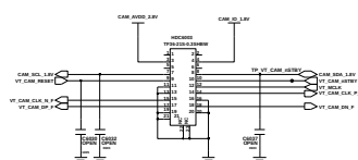
2M CAM
